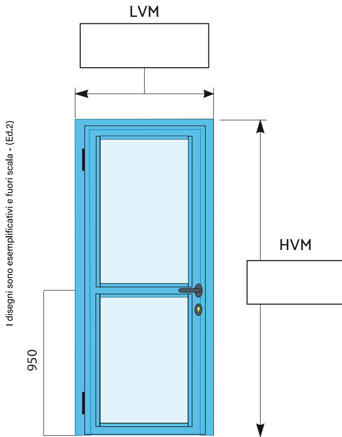
Porta finestra con fermavetri "lato a tirare"
